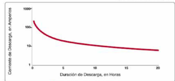
CAPACIDAD DE RESERVA SEGÚN DESCARGA
