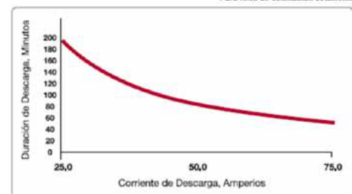
CAPACIDAD DE RESERVA SEGÚN DESCARGA
